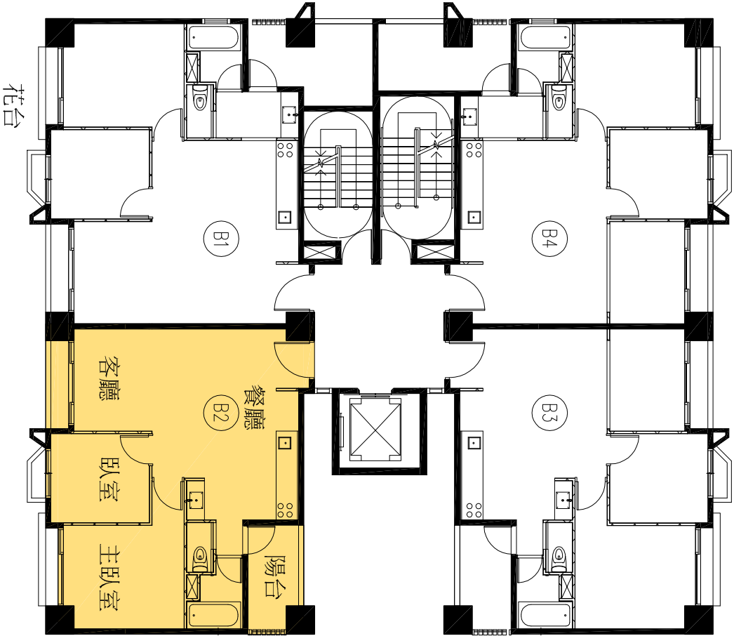
標準戶B2平面配置圖
