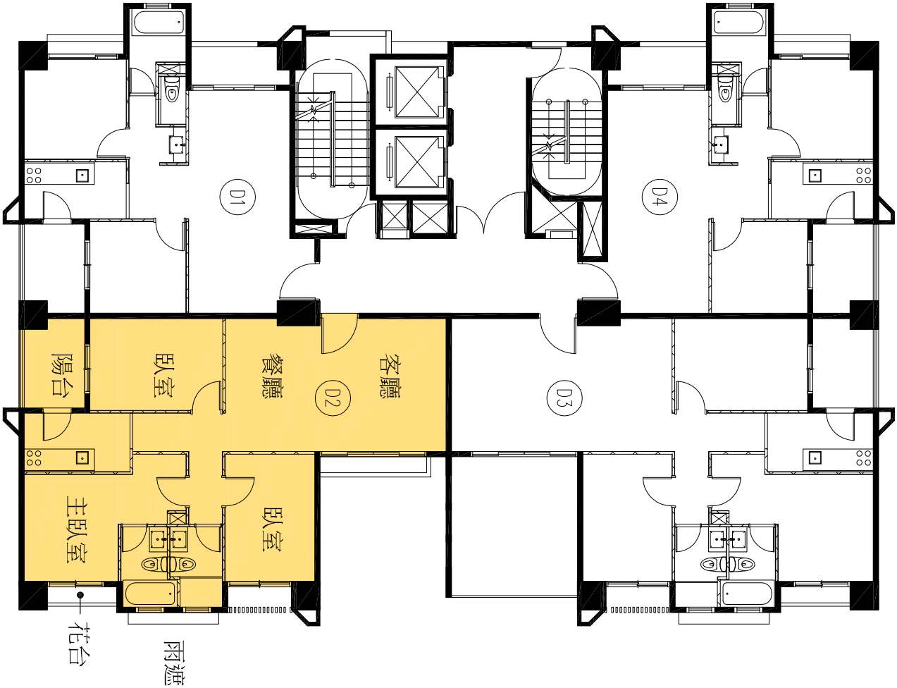
標準戶D2平面配置圖(單數層)
