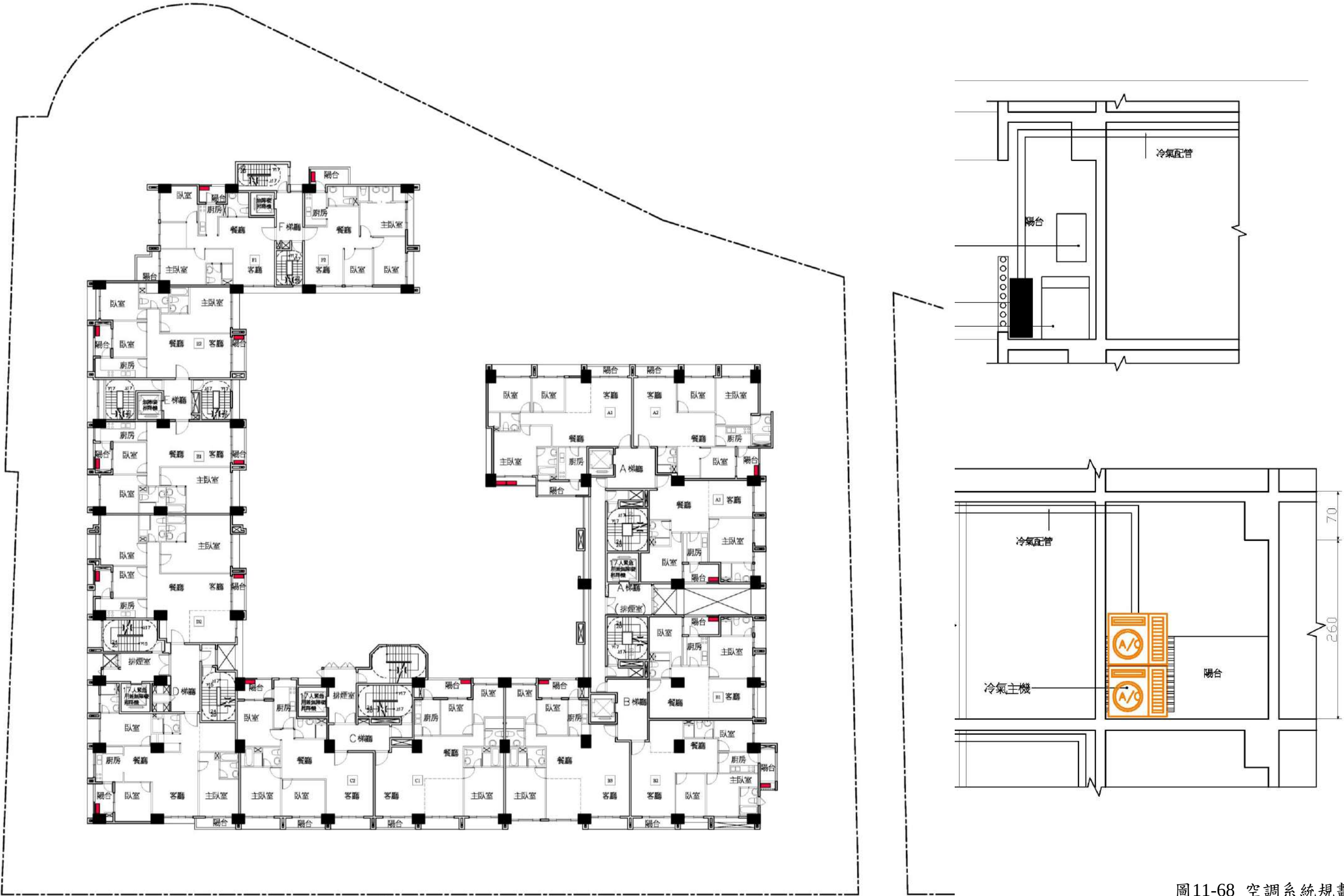
圖11-68 空調系統規劃圖
