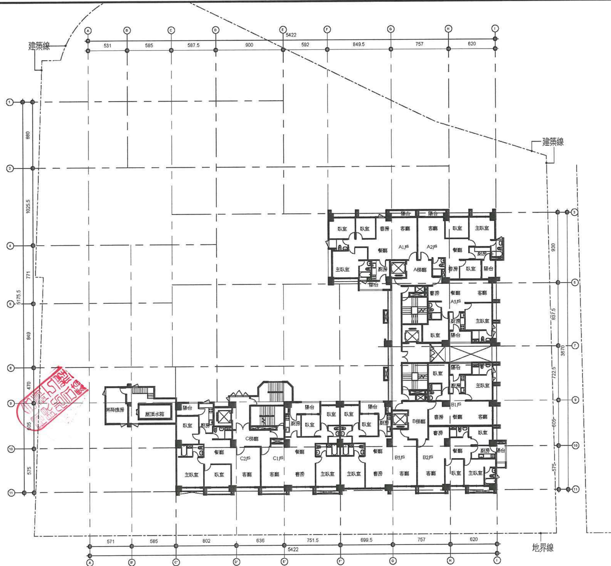
圖6-40 二十一層平面圖(S=1/300)
