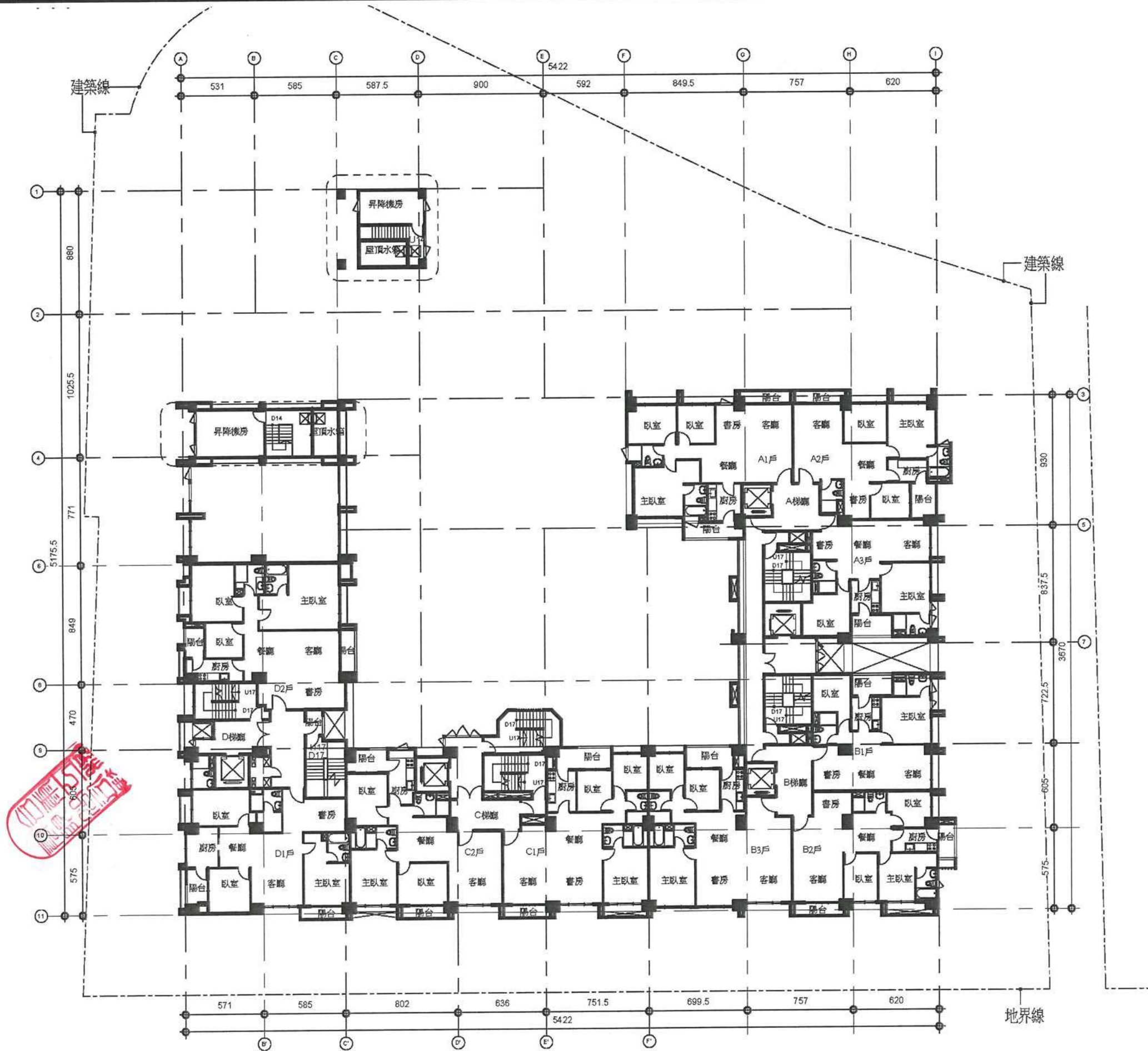
圖6-34 十五層平面圖(S=1/300)
