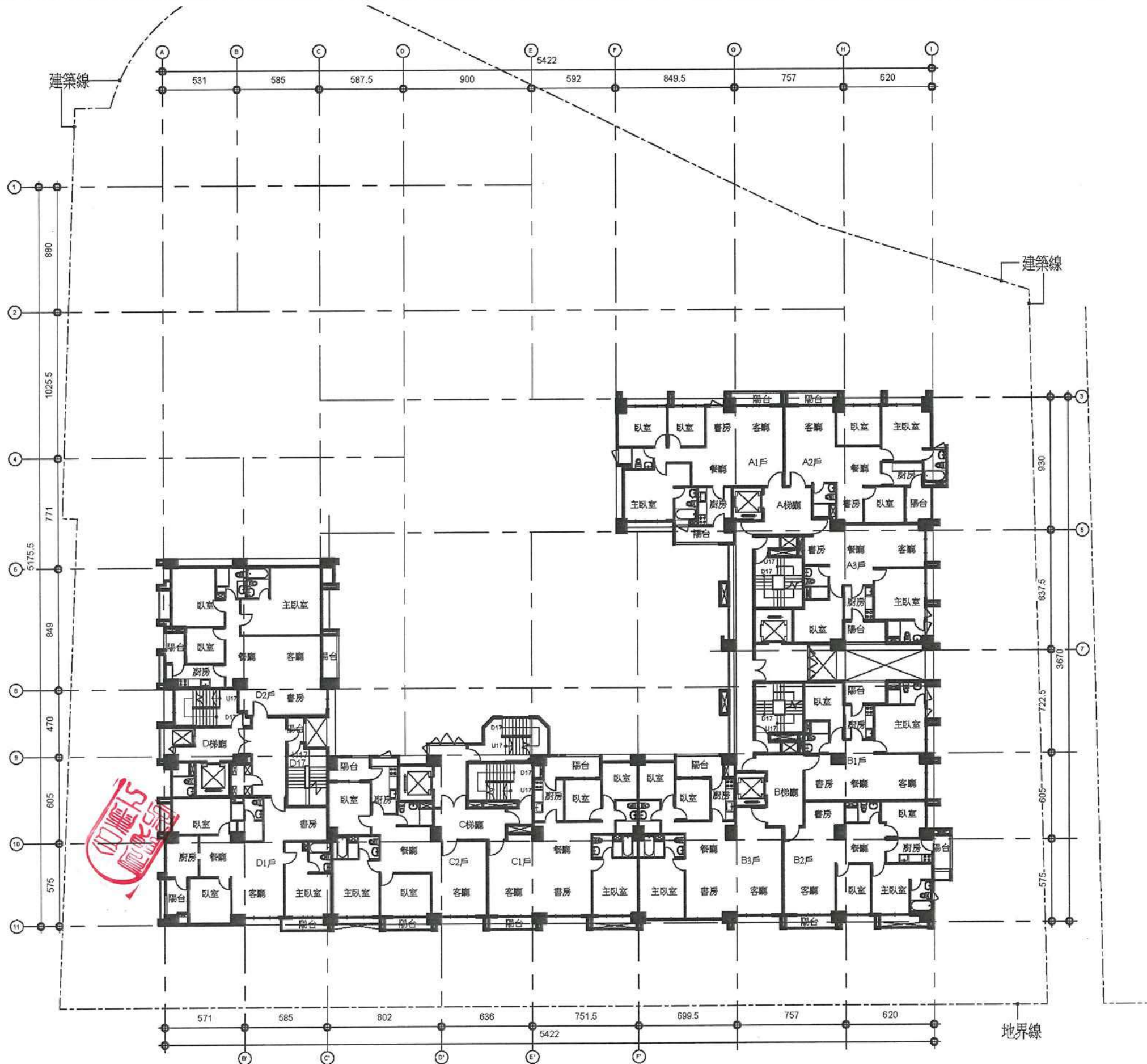
圖6-36 十七、十九層平面圖(S=1/300)
