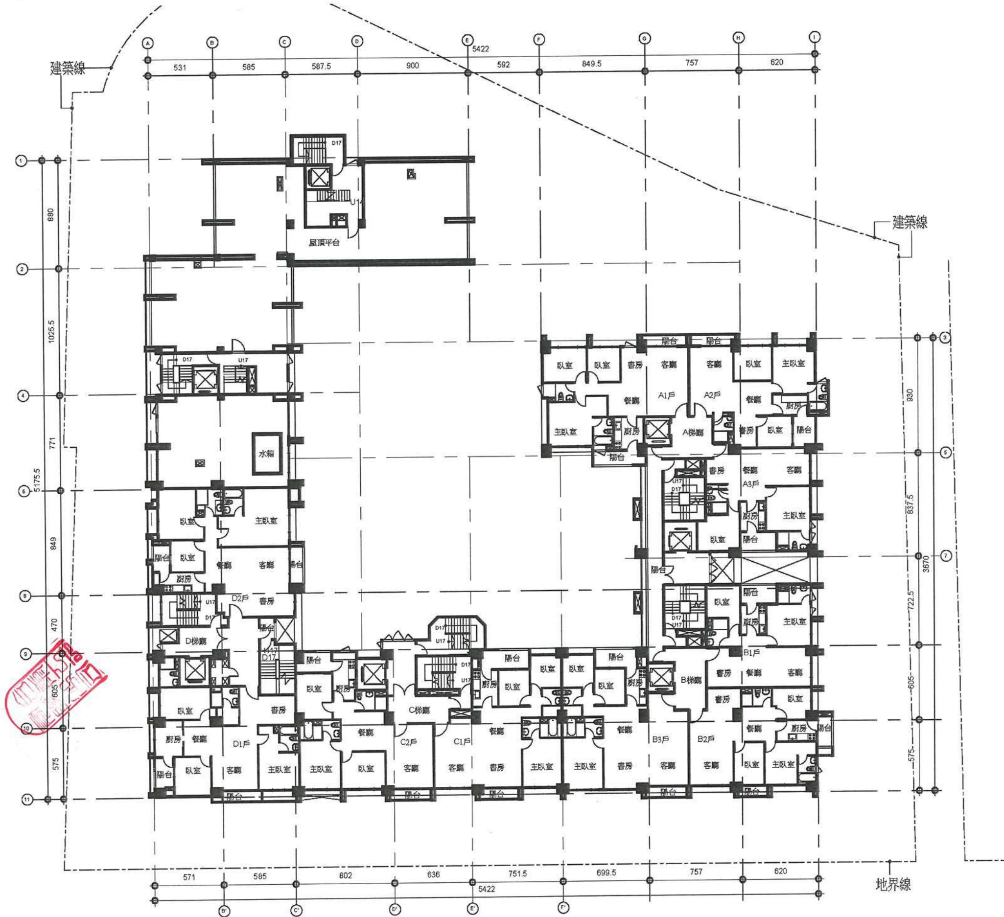
圖6-32 十四層平面圖(S=1/300)
