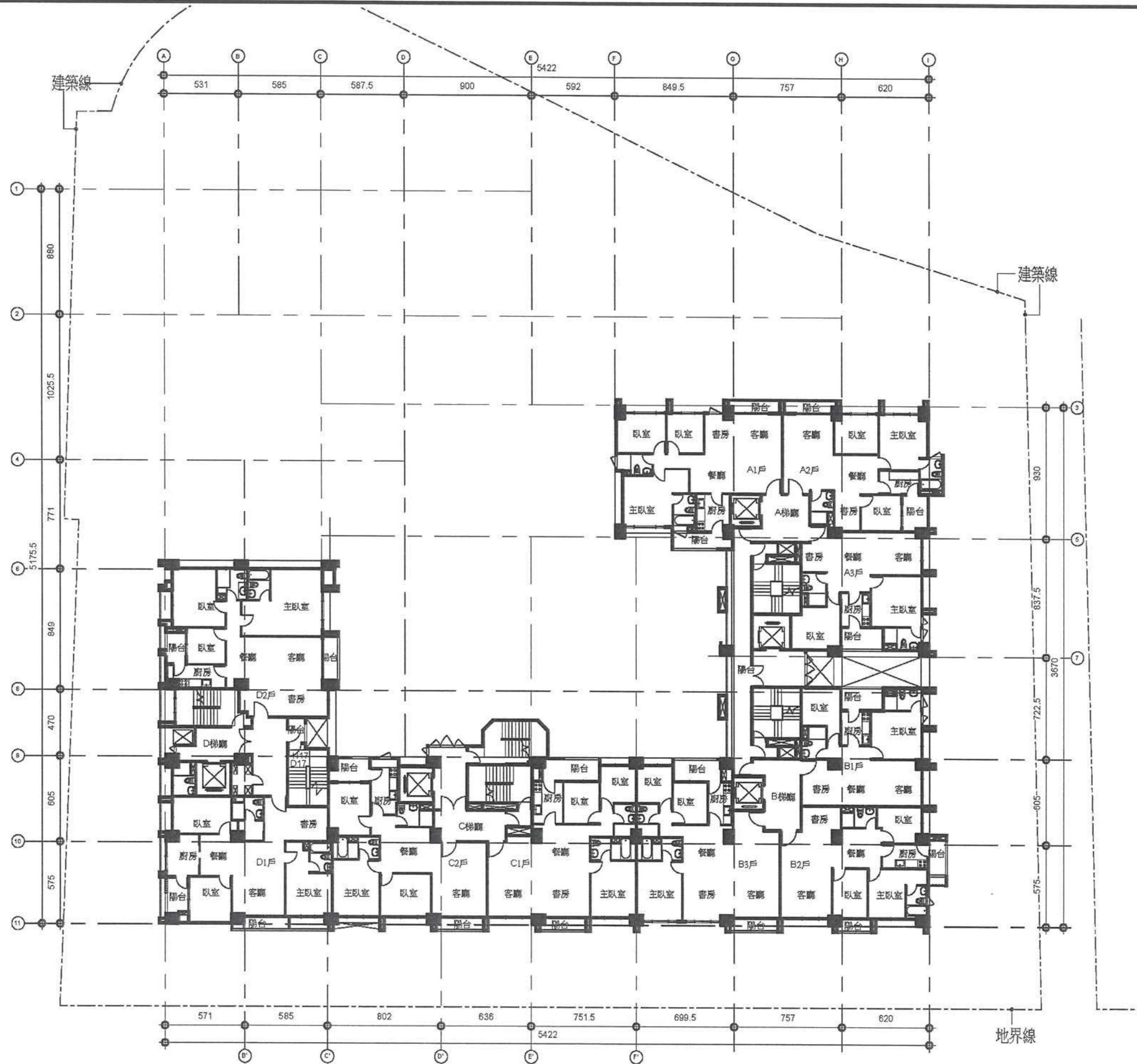
圖6-35 十六、十八層平面圖(S=1/300)
