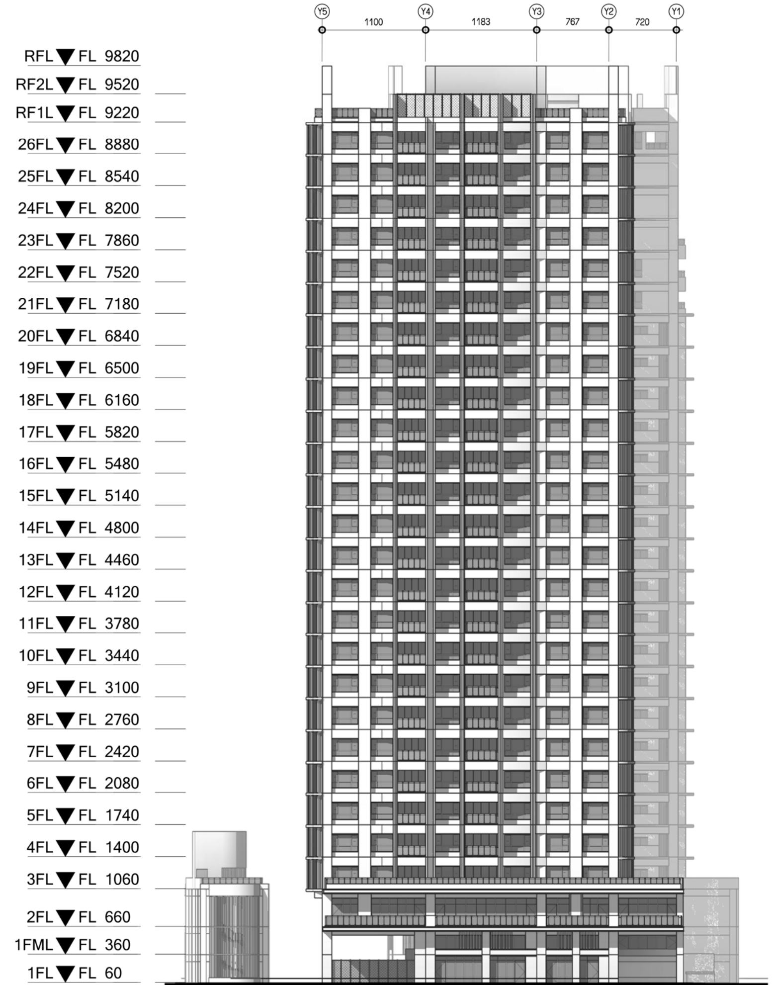
東向立面圖 SCALE:1/400 P.3-14
