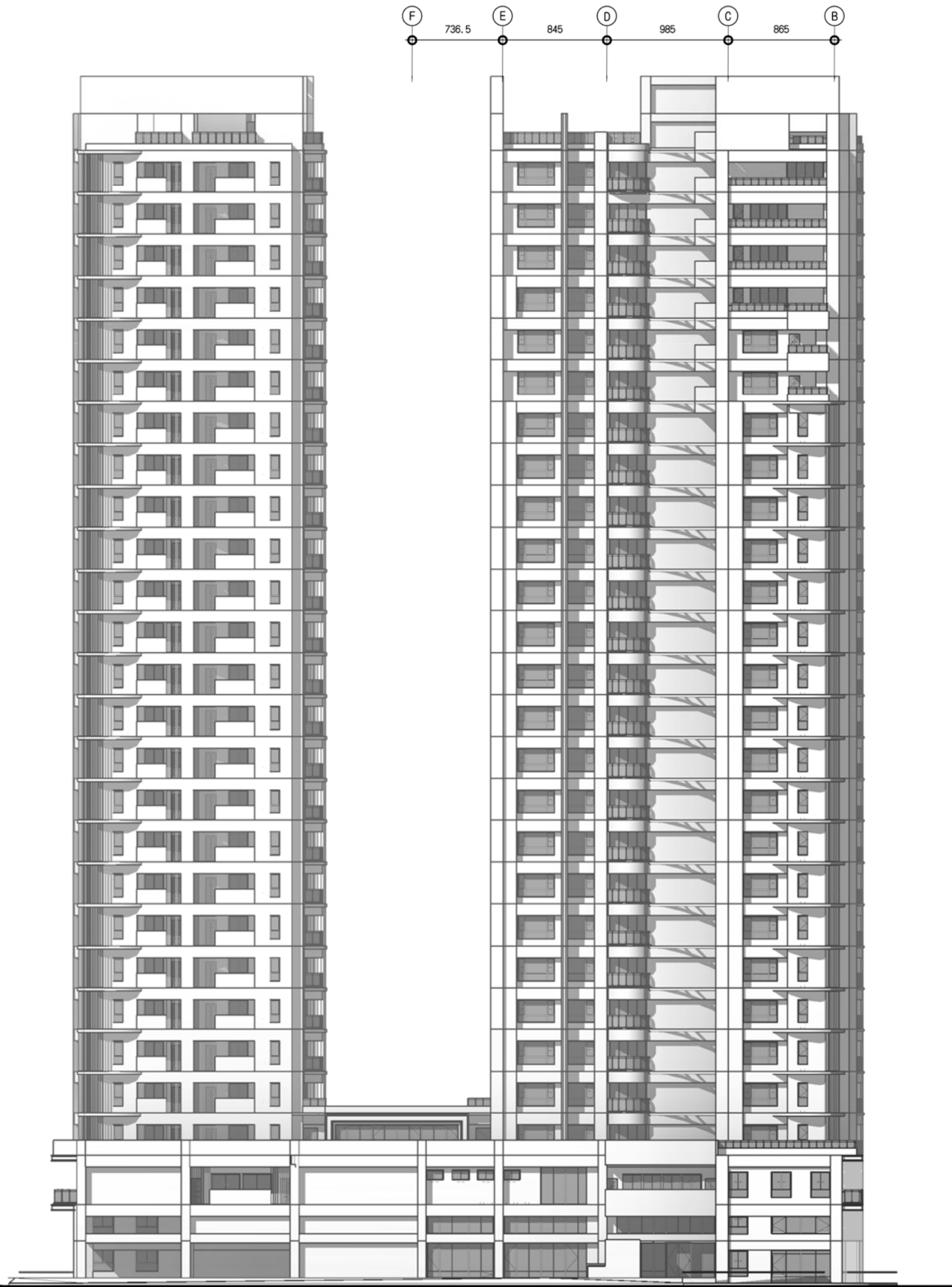
北向立面圖 SCALE:1/400
