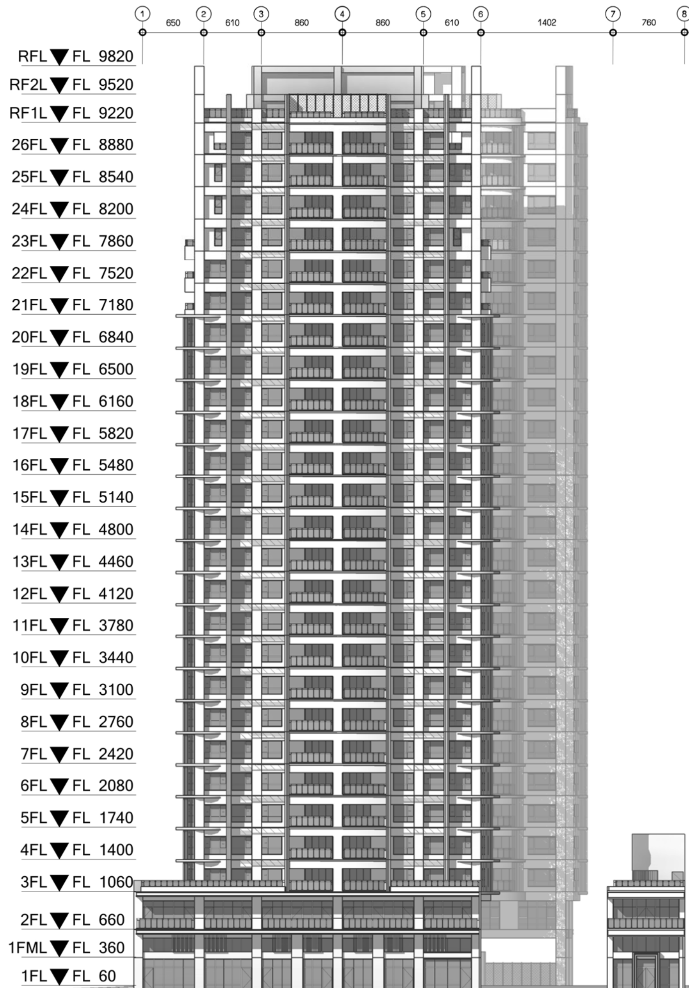
西向立面圖 SCALE:1/400
