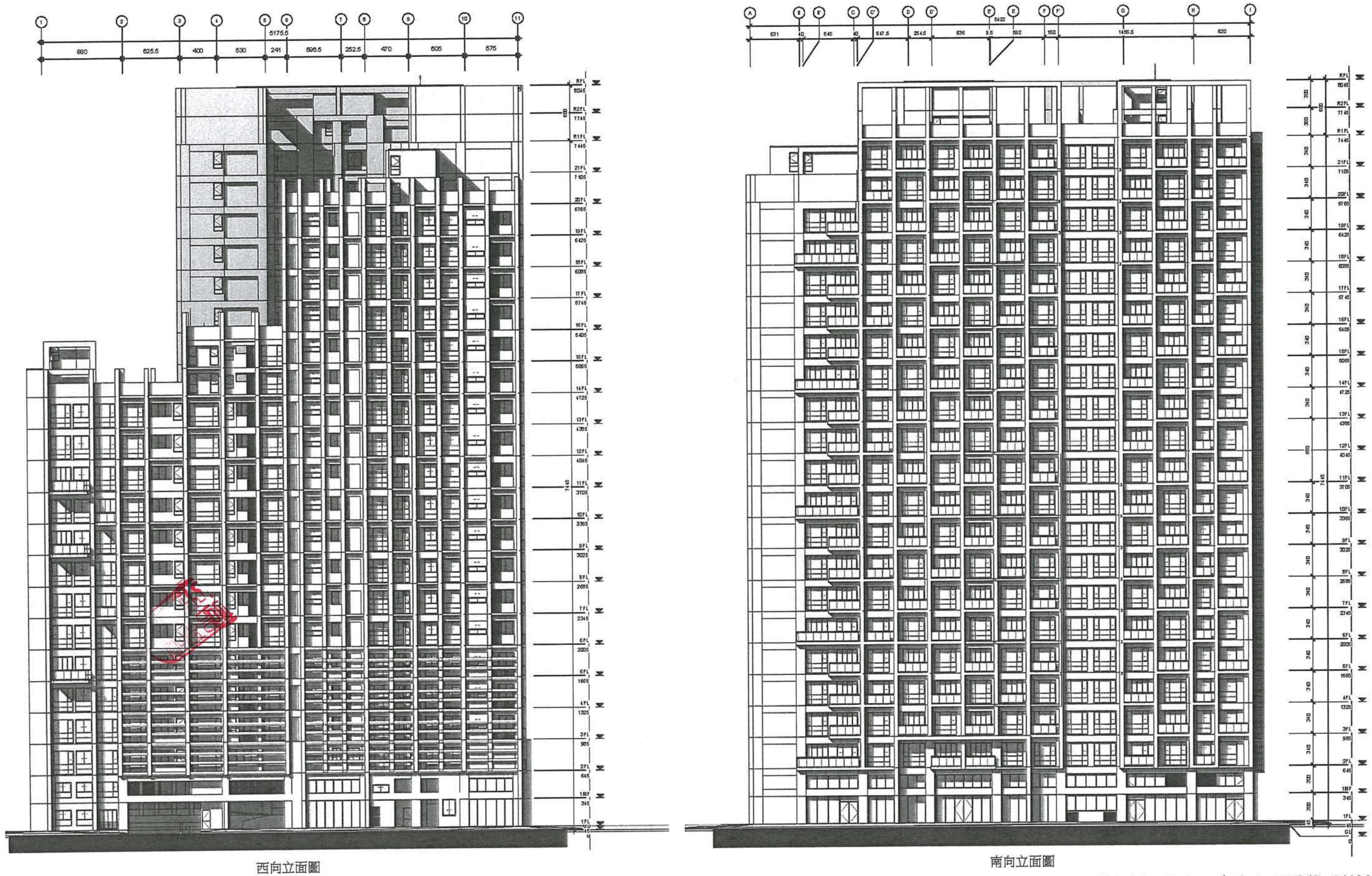
圖6-44 西向、南向立面圖(S=1/400)
