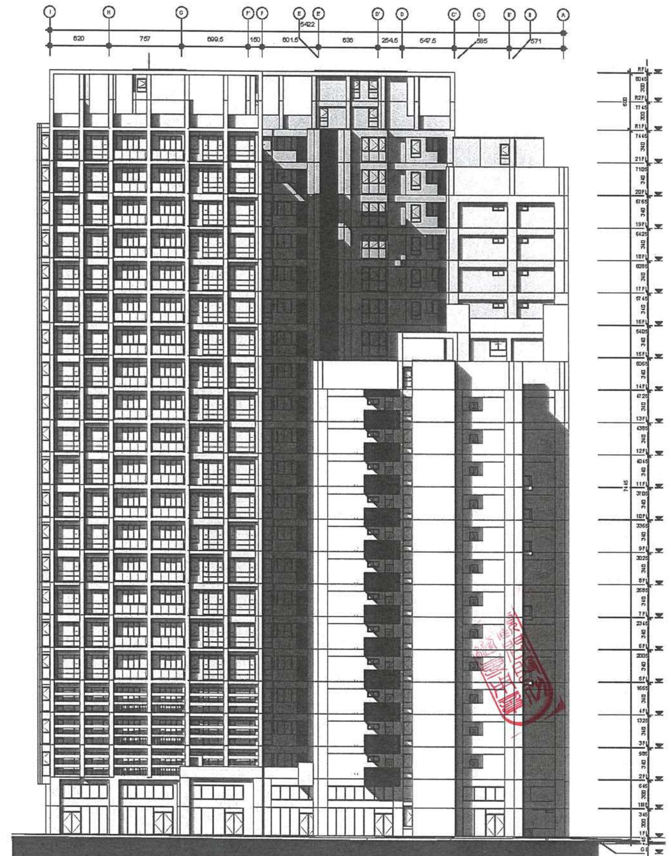
北向立面圖
