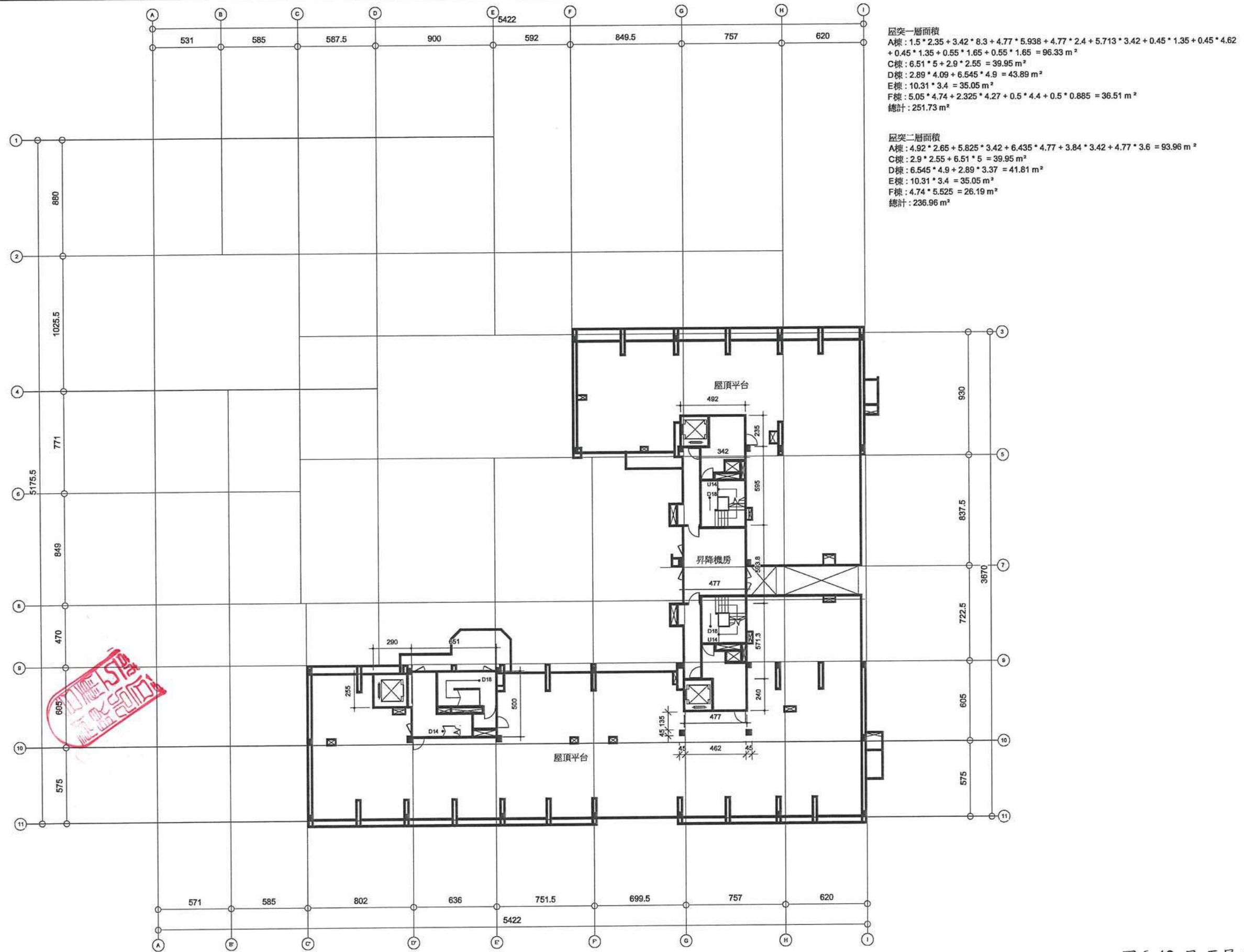
圖6-42 屋頂層平面圖(S=1/300)
