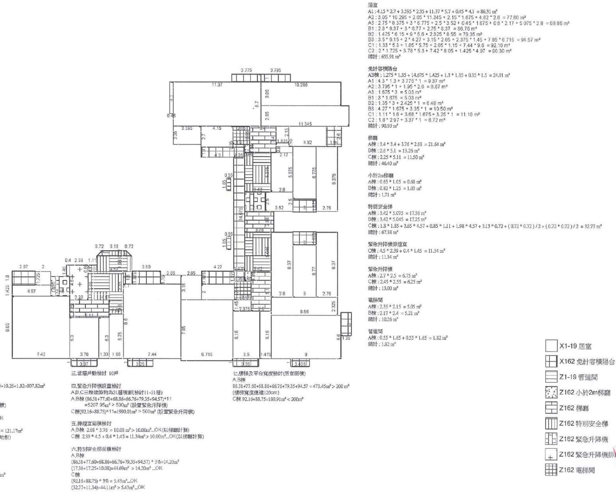
圖11-40 二十層面積計算圖(S=1/300)
