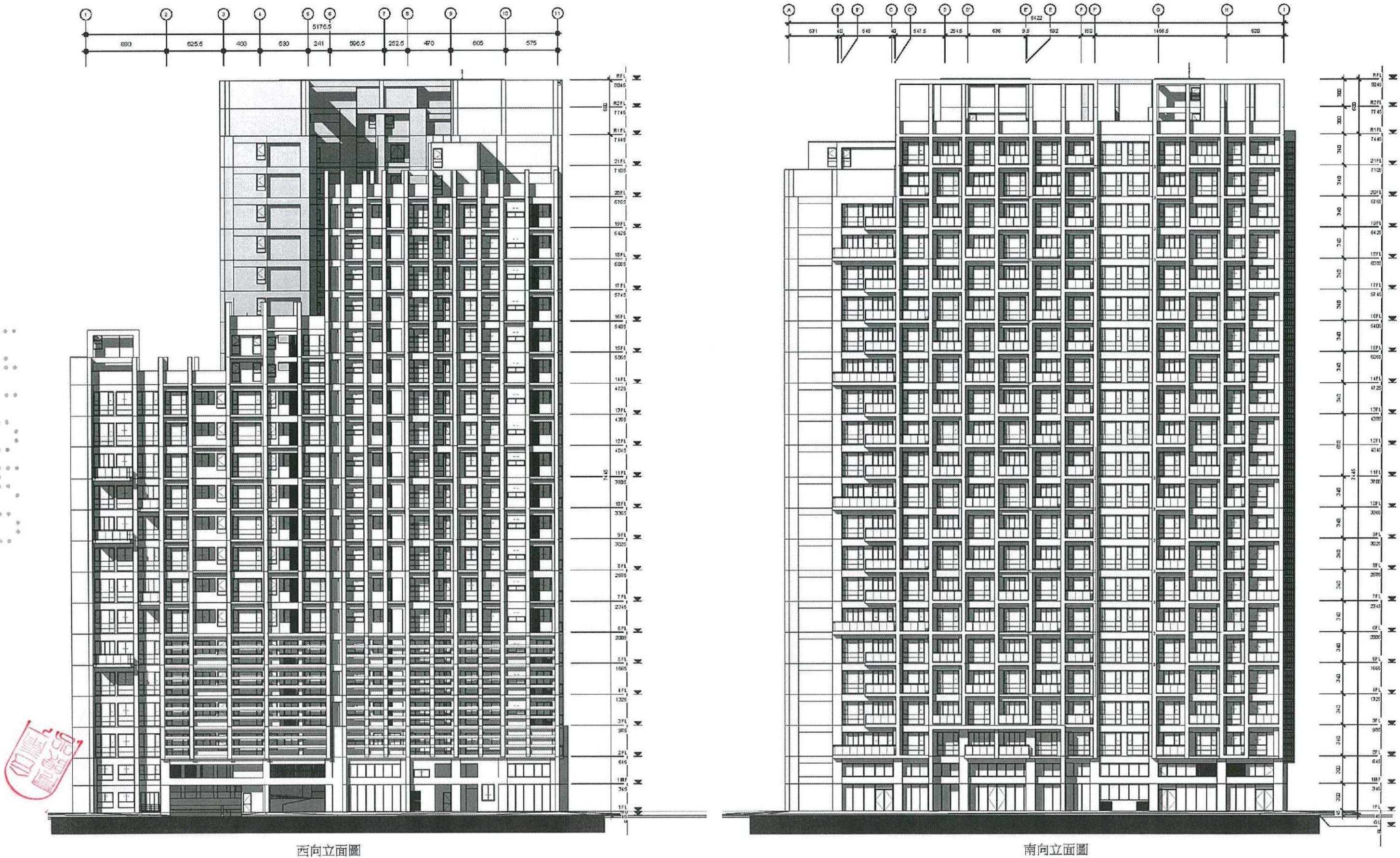
圖11-45 西向、南向立面圖(S=1/400)
