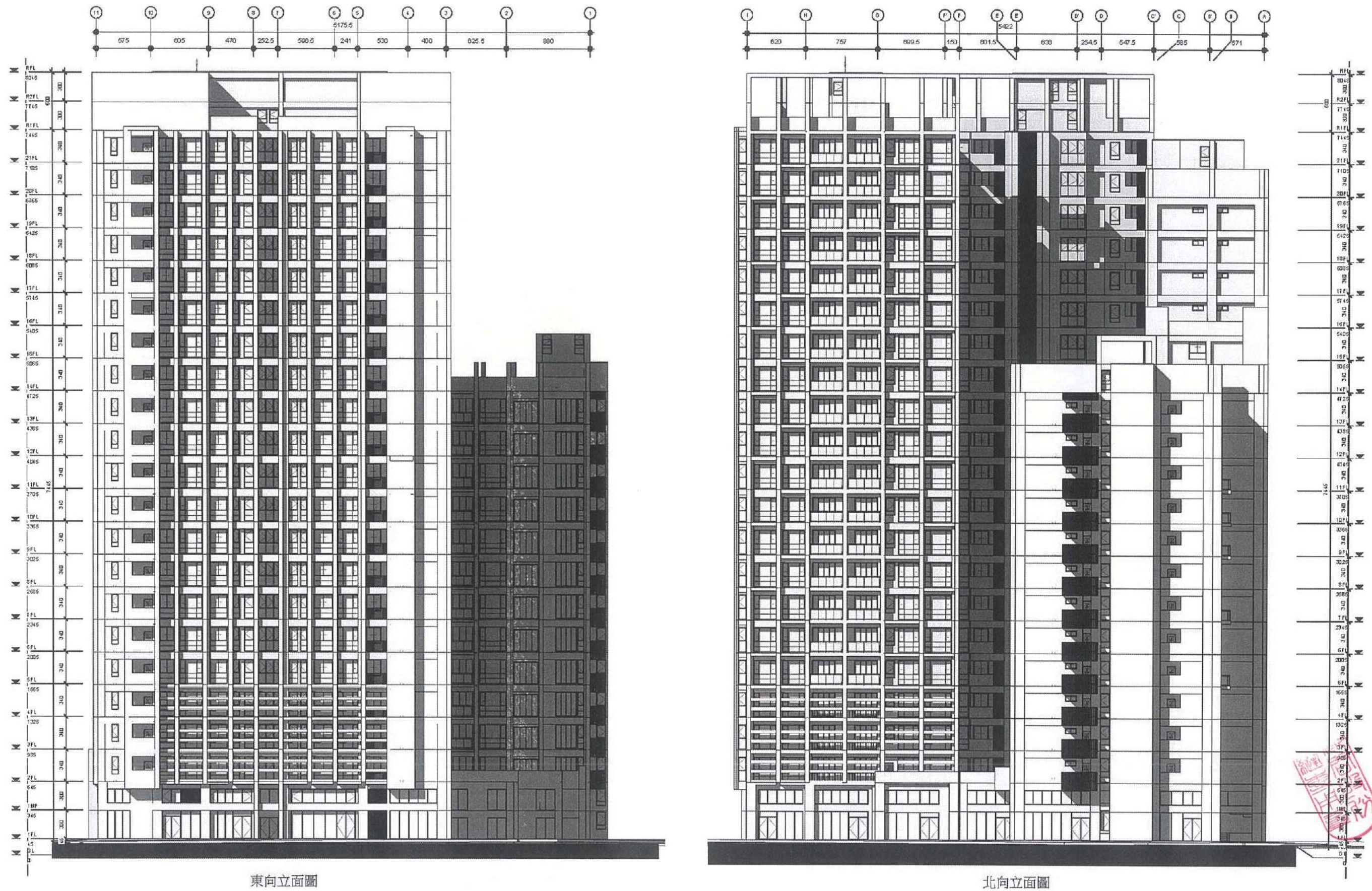
圖11-44 東向、北向立面圖(S=1/400)
