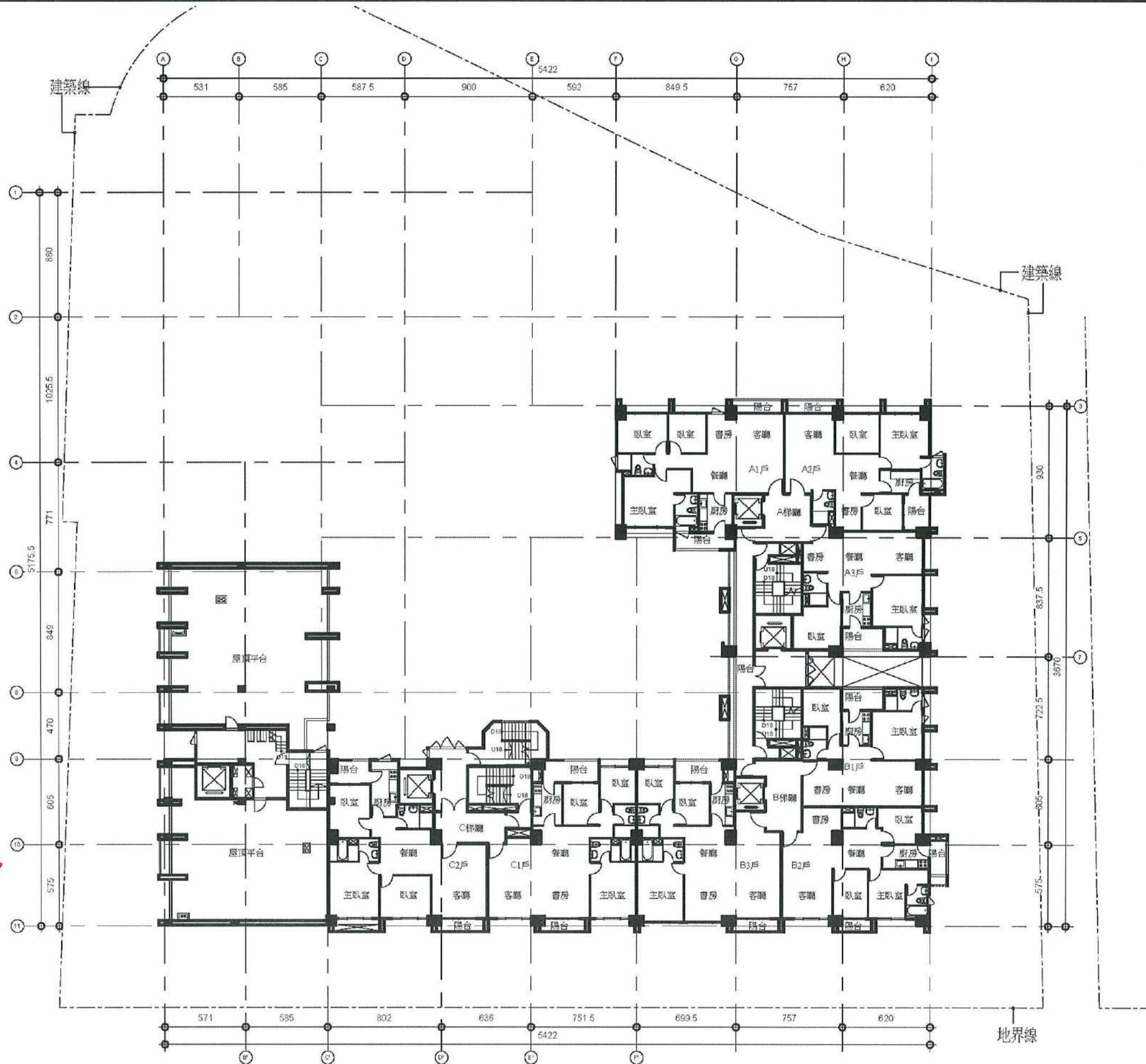
圖11-39 二十層平面圖(S=1/300)
