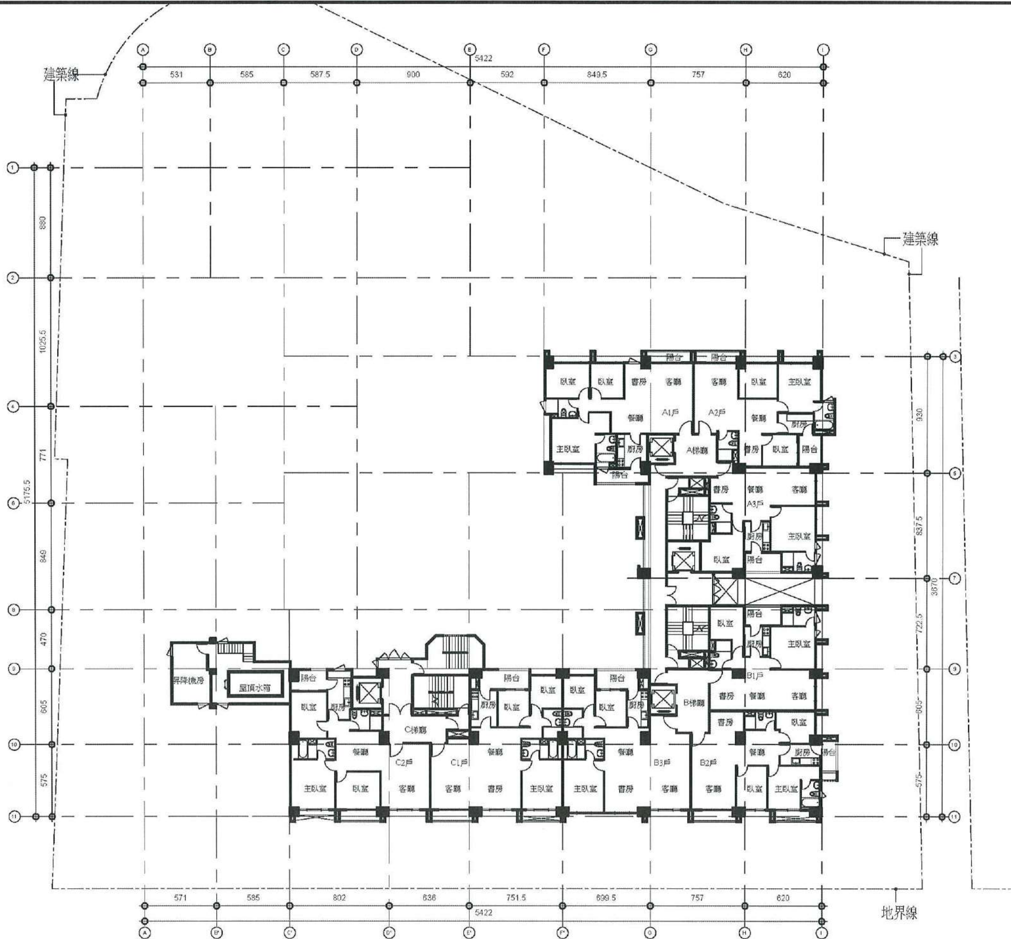
圖11-41 二十一層平面圖(S=1/300)
